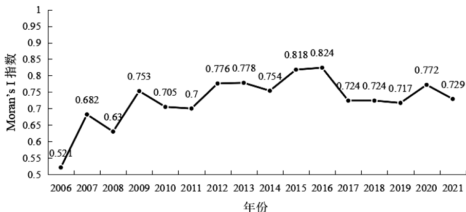
图 4 长江经济带物流效率全局空间自相关系数 Global Moran's I
